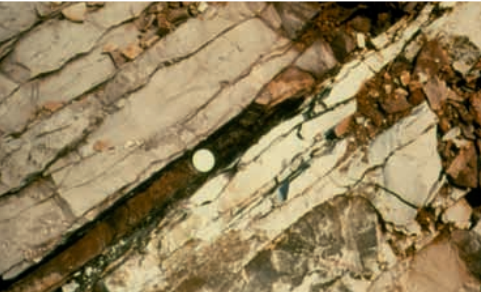
A fronteira K/T, uma camada preta entre as rochas cretácea e terciária, é constituída de material liberado pelo impacto de um asteróide.
