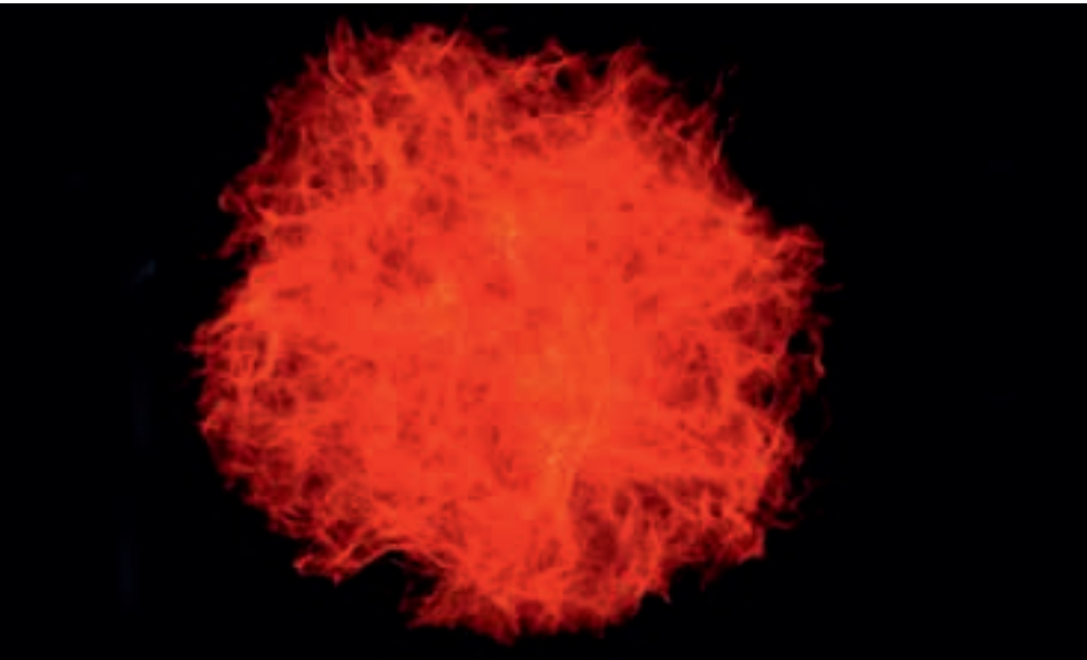
Uma ilustração conceitual da explosão, feita por computador, mostra a expansão de gás e matéria que iria se tornar o nosso universo.
